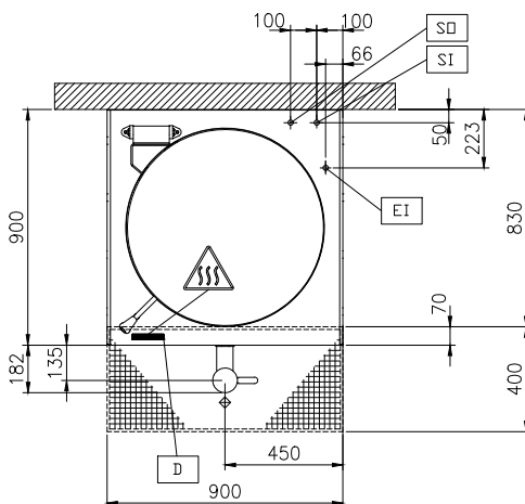
Boven aanzicht
